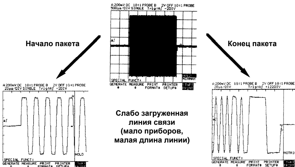
Рисунок 33 Типичная осциллограмма сигнала при слабой загрузке линии связи
